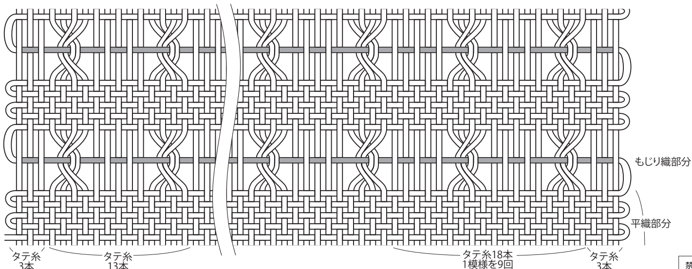
〈もじり織デザイン図〉
